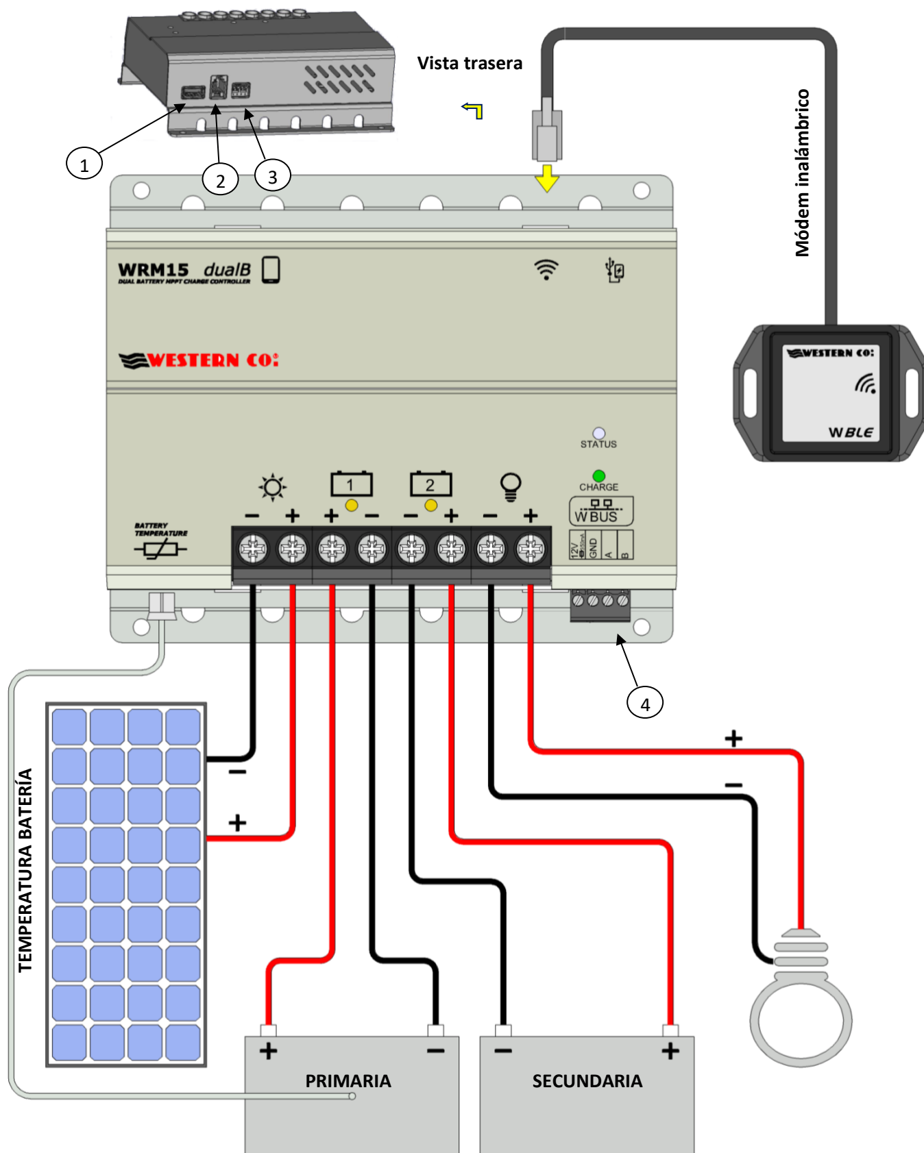
Fig. 2. Esquema de conexión
