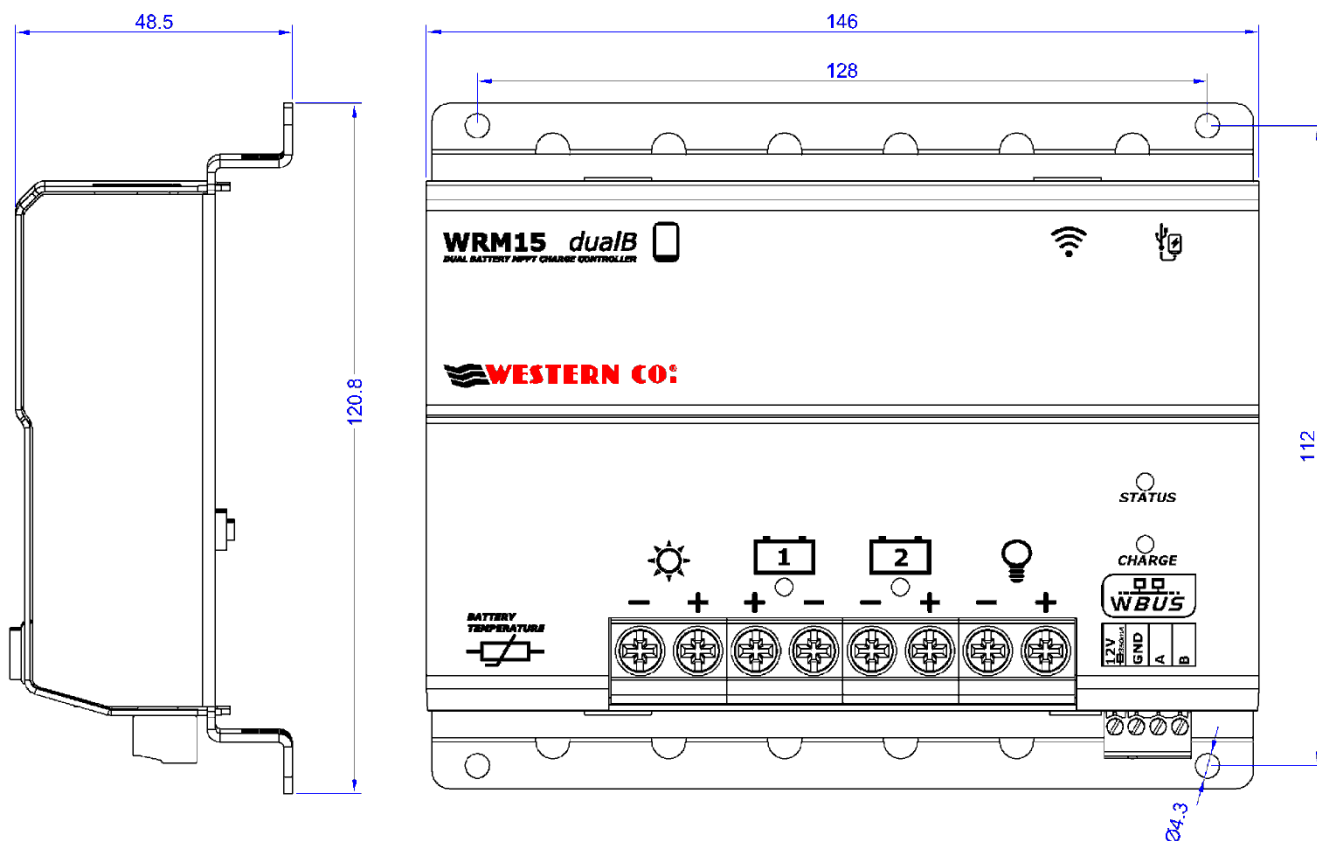
Fig. 5 Dimesions (mm)
