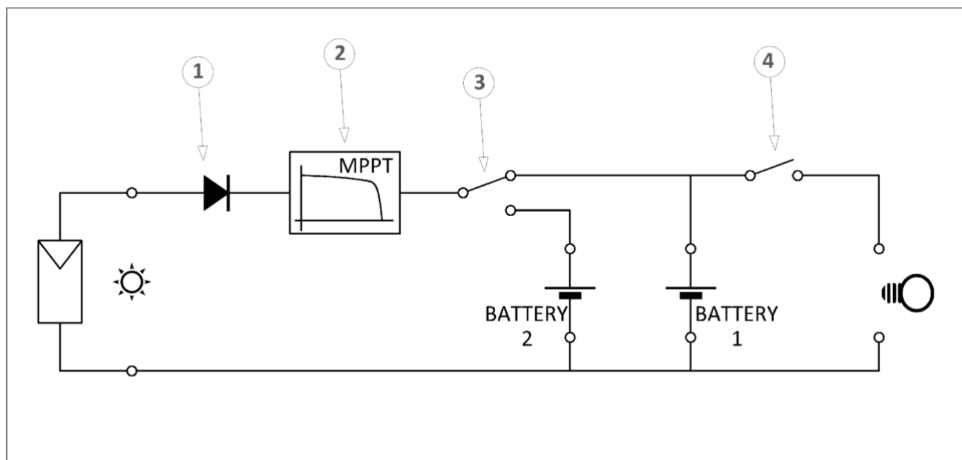
Fig. 1. Esquema de principio
