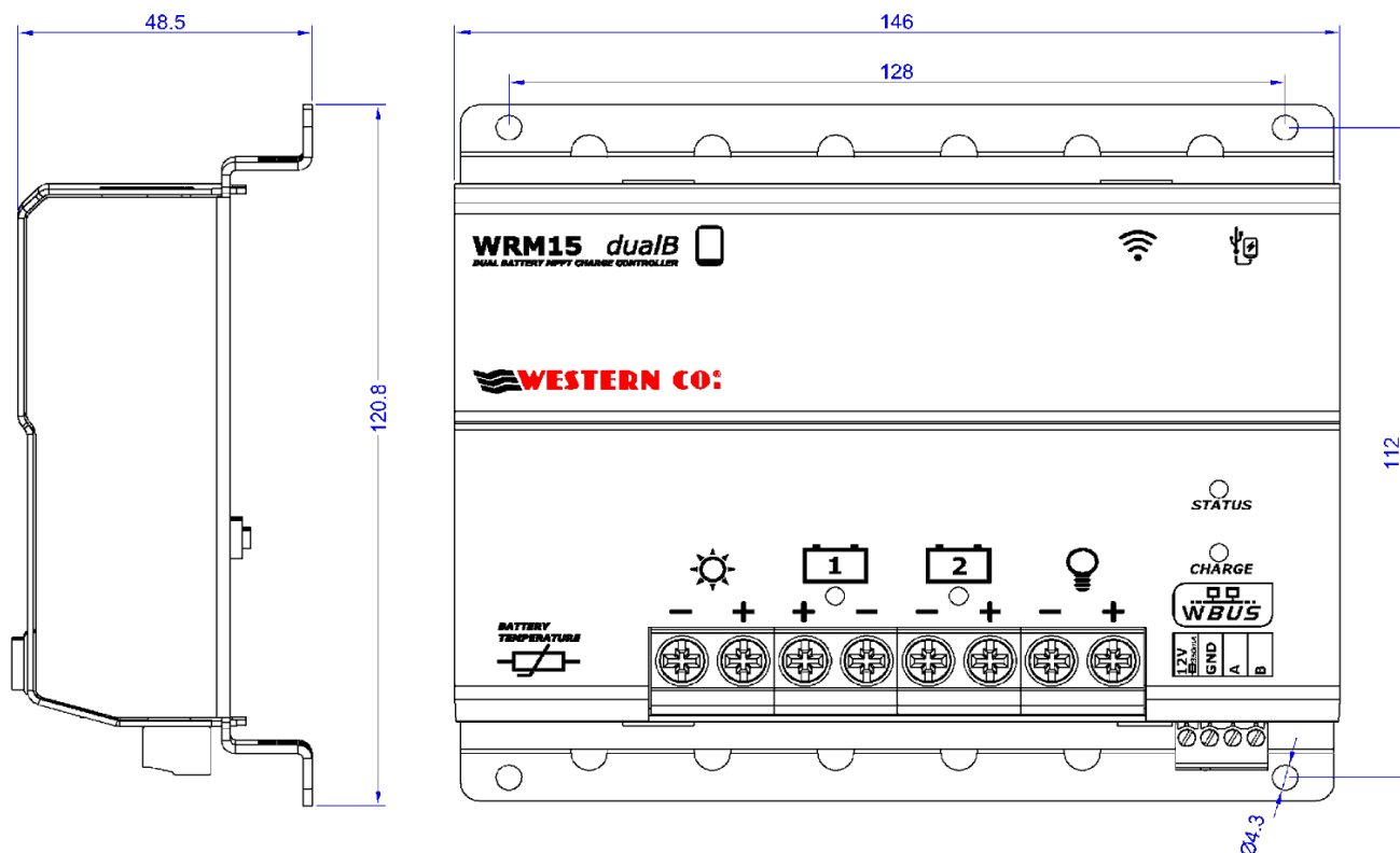
Fig. 5 Dimensioni (mm)
