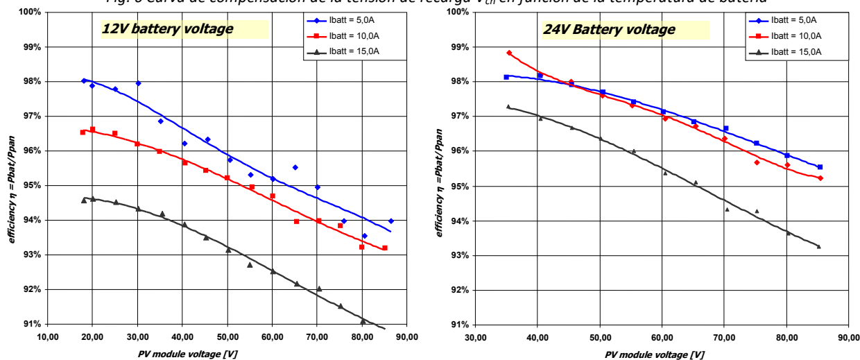
Fig. 7 Rendimiento del WRM15 dualB/dualB-E en función de la tensión de panel para sistema de 12 V y 24 V
